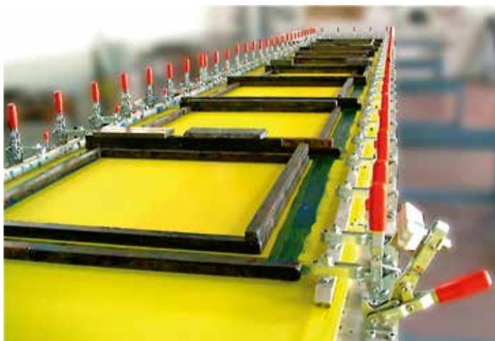
Rahmenprofile müssen im rechten Winkel stehen und so planparallel wie möglich liegen, da ansonsten später kein homogenes Siebspannergebnis möglich ist. (Foto: Tiflex)
