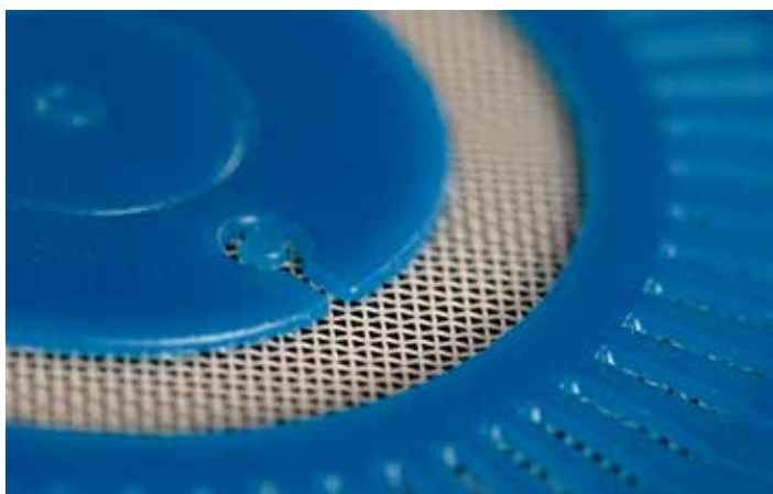
Dickschicht-Schablone mit einer hochviskosen Kopierschicht (Foto: Kissel+Wolf)
